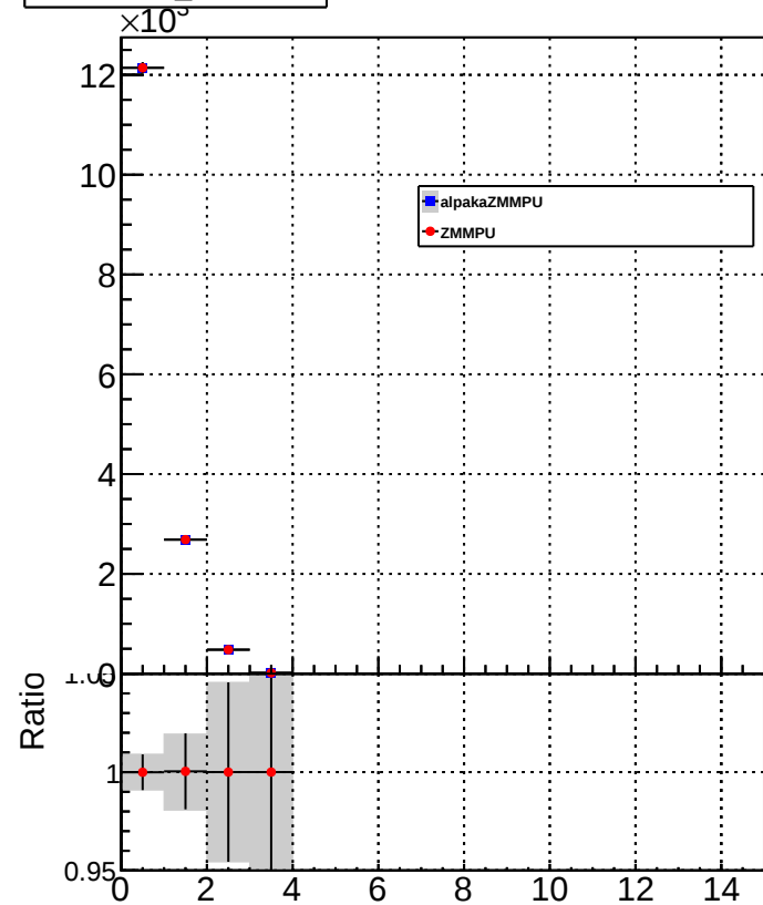
NJetsEta_E 40<Pt
