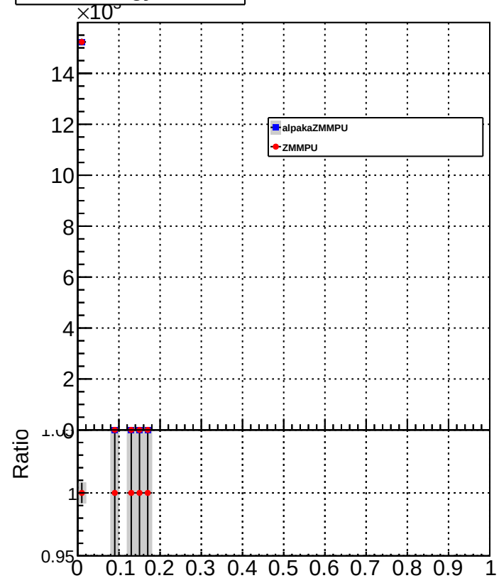
HFEMEnergyFraction
