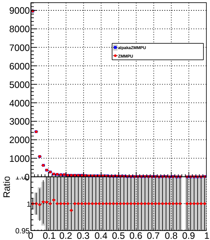
neutralEmEnergyFraction
