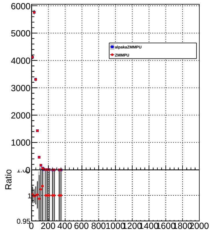
MET (20 GeV binning)
