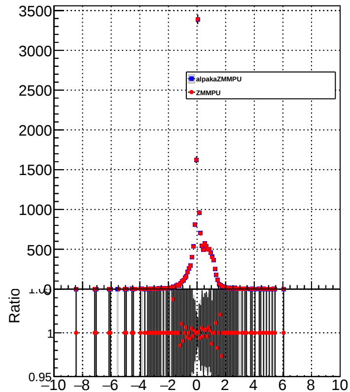
METUnc_TauEnDown
