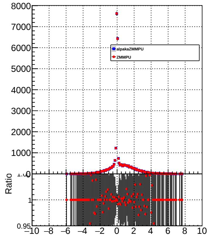
METUnc_UnclusteredEnDown
