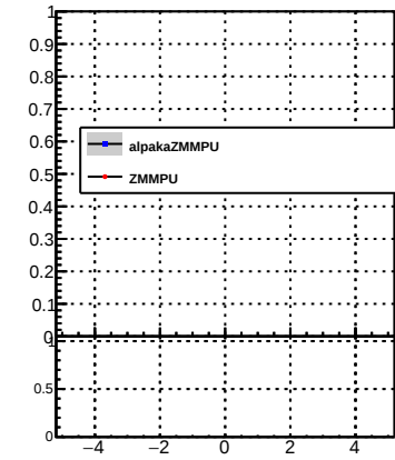
p_offset_eta_npv21_nh
