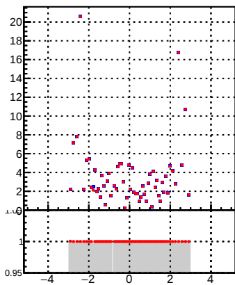
p_offset_eta_npv23_chu
