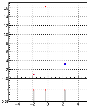
p_offset_eta_npv23_lep
