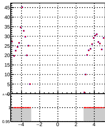
p_offset_eta_npv23_hfh
