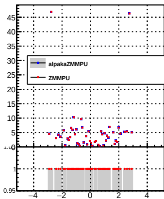
p_offset_eta_npv23_nh
