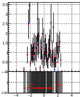
p_offset_eta_npv34_lep
