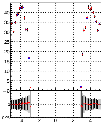
p_offset_eta_npv34_hfh
