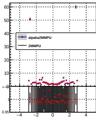
p_offset_eta_npv34_nh
