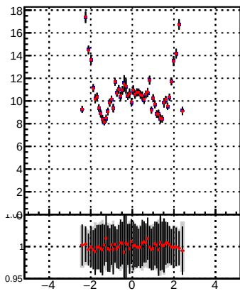
p_offset_eta_npv34_chm
