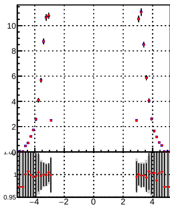
p_offset_eta_npv34_hfe
