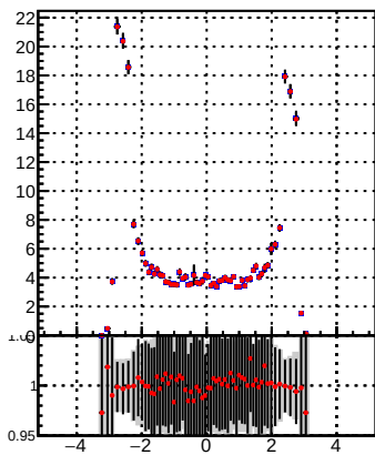
p_offset_eta_npv34_chu
