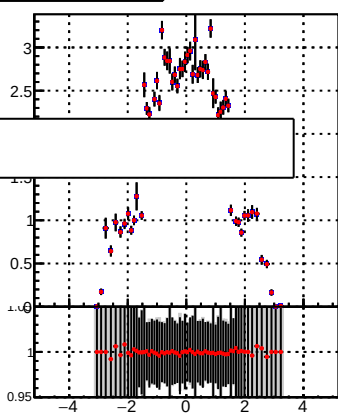
p_offset_eta_npv39_ne
