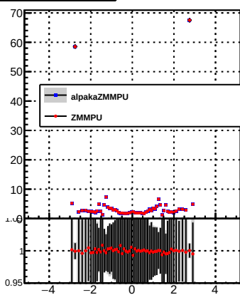
p_offset_eta_npv39_nh
