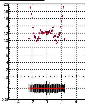
p_offset_eta_npv39_chm
