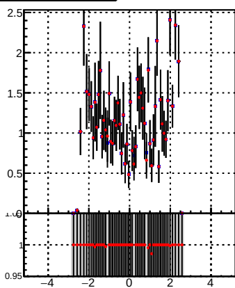
p_offset_eta_npv39_lep
