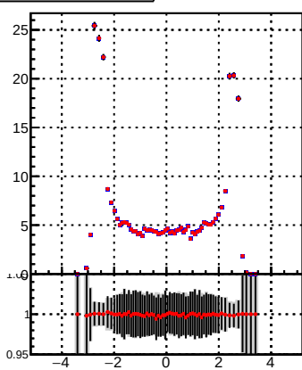
p_offset_eta_npv39_chu
