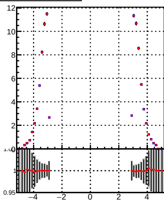
p_offset_eta_npv39_hfe
