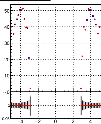
p_offset_eta_npv39_hfh
