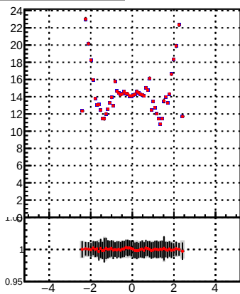
p_offset_eta_npv48_chm
