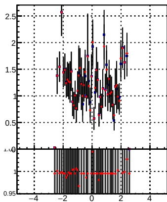
p_offset_eta_npv57_lep
