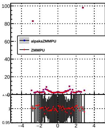
p_offset_eta_npv57_nh
