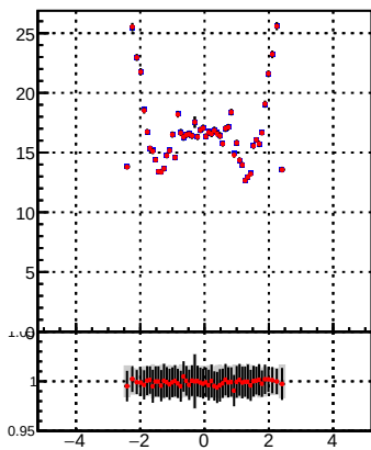
p_offset_eta_npv57_chm
