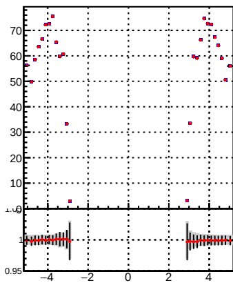
p_offset_eta_npv57_hfh
