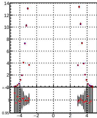
p_offset_eta_npv57_hfe
