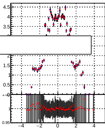
p_offset_eta_npv57_ne
