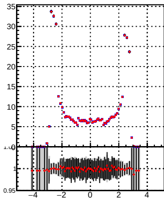
p_offset_eta_npv57_chu
