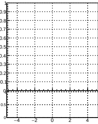
p_offset_eta_npv82_chm
