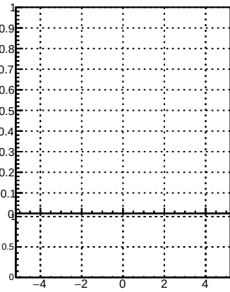
p_offset_eta_npv82_lep
