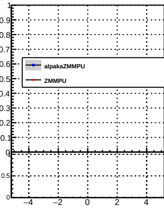
p_offset_eta_npv82_nh
