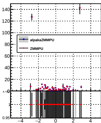
p_offset_eta_npv84_nh
