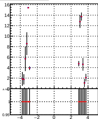
p_offset_eta_npv84_hfe
