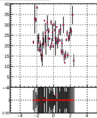
p_offset_eta_npv84_chm
