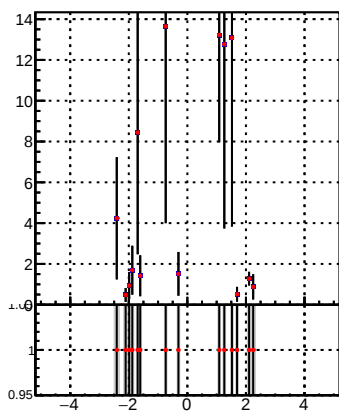
p_offset_eta_npv84_lep
