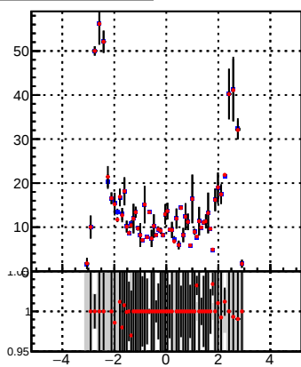
p_offset_eta_npv84_chu
