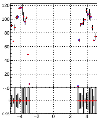
p_offset_eta_npv84_hfh
