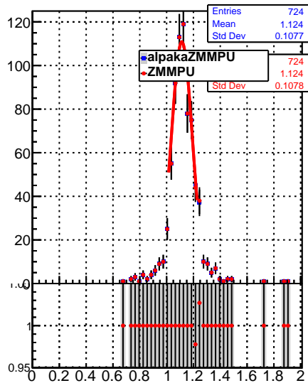
Raw Jet response (pT/pTgen) in 49 &lt;math&gt;=&lt;/math&gt; pt &lt;math&gt;&lt; 64, 0.0 &lt;= &lt;/math&gt; |eta| &lt;math&gt;&lt; 0.5&lt;/math&gt;
