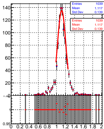
Raw Jet response (pT/pTgen) in 49 &lt;math&gt;=&lt;/math&gt; pt &lt;math&gt;&lt; 64, 1.3 &lt;= &lt;/math&gt; |eta| &lt;math&gt;&lt; 2.1&lt;/math&gt;
