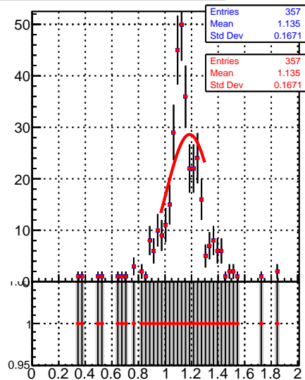
Raw Jet response (pT/pTgen) in 49 &lt;math&gt;=&lt;/math&gt; pt &lt;math&gt;&lt; 64, 2.1 &lt;= &lt;/math&gt; |eta| &lt;math&gt;&lt; 2.5&lt;/math&gt;
