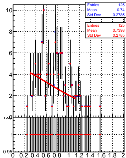
Raw Jet response (pT/pTgen) in 49 &lt;math&gt;=&lt;/math&gt; pt &lt;math&gt;&lt; 64, 2.5 &lt;= &lt;/math&gt; |eta| &lt;math&gt;&lt; 3.0&lt;/math&gt;
