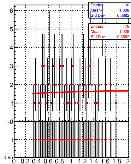
Raw Jet response (pT/pTgen) in 49 &lt;math&gt;=&lt;/math&gt; pt &lt;math&gt;&lt; 64, 3.0 &lt;= &lt;/math&gt; |eta| &lt;math&gt;&lt; 5.0&lt;/math&gt;
