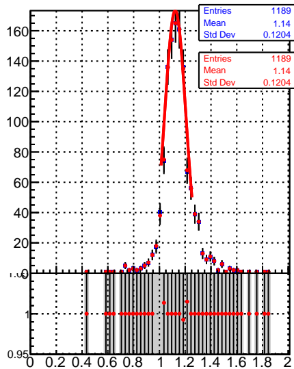
Raw Jet response (pT/pTgen) in 49 &lt;math&gt;=&lt;/math&gt; pt &lt;math&gt;&lt; 64, 0.5 &lt;= &lt;/math&gt; |eta| &lt;math&gt;&lt; 1.3&lt;/math&gt;
