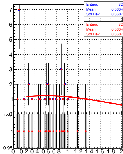
Raw Jet response (pT/pTgen) in 64 &lt;math&gt;pt &lt; 84, 3.0 &lt;= |\eta| &lt; 5.0&lt;/math&gt;
