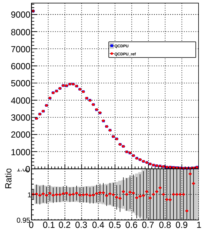
neutralEmEnergyFraction
