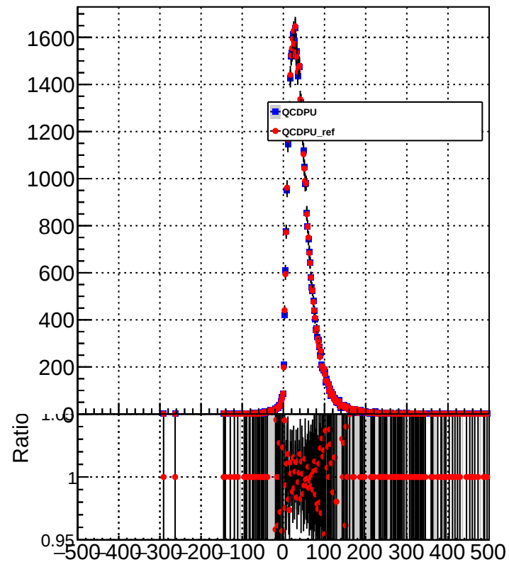
METDifference_GenMETTrue
