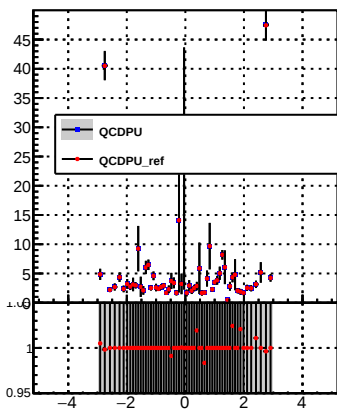
p_offset_eta_npv26_nh
