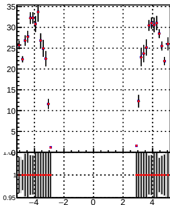
p_offset_eta_npv26_hfh
