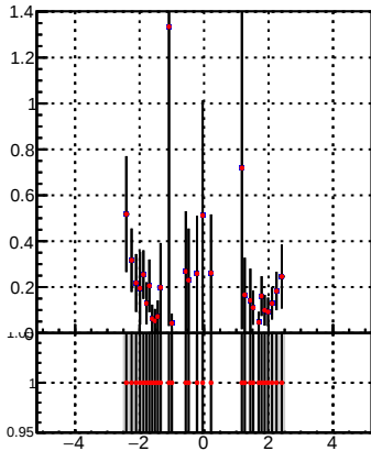
p_offset_eta_npv26_lep
