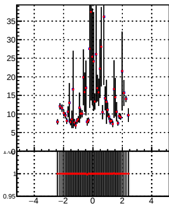
p_offset_eta_npv26_chm
