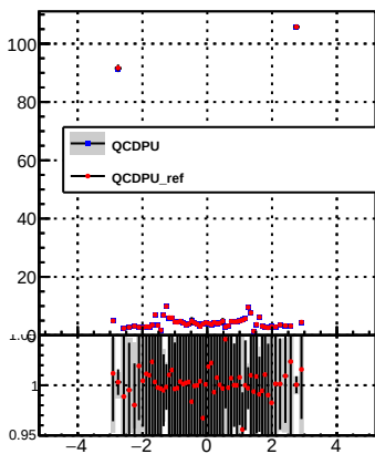
p_offset_eta_npv59_nh
