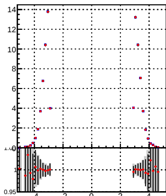
p_offset_eta_npv59_hfe
