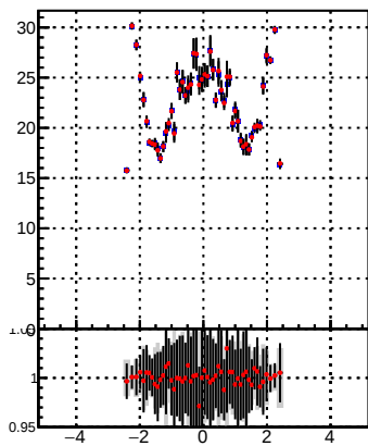
p_offset_eta_npv59_chm
