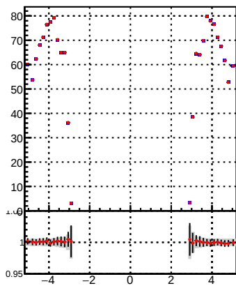
p_offset_eta_npv59_hfh
