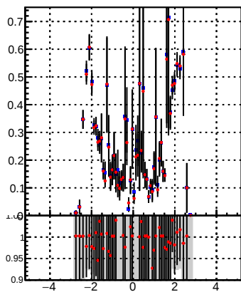
p_offset_eta_npv59_lep
