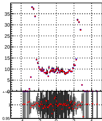
p_offset_eta_npv59_chu
