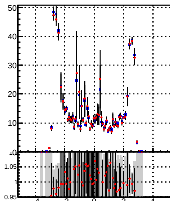
p_offset_eta_npv74_chu
