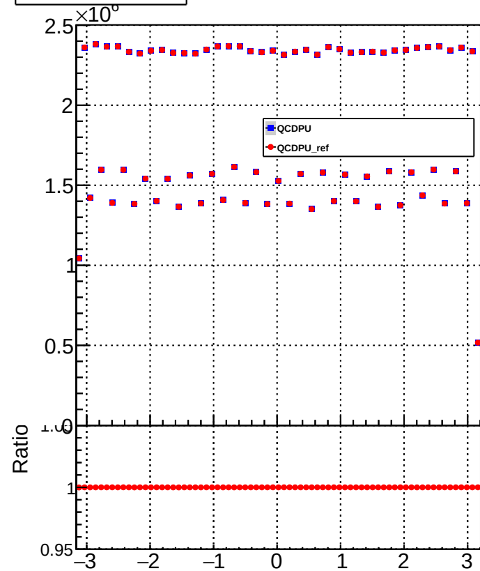
AllCandidatePhi
