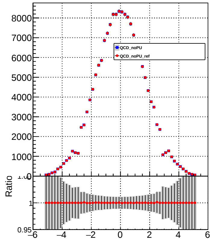
CorrJetEta Pt&gt;20
