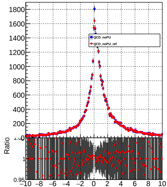
METUnc_JetEnDown
