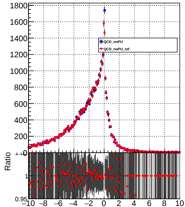
METUnc_JetResUp
