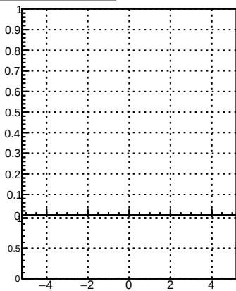
p_offset_eta_npv46_hfe
