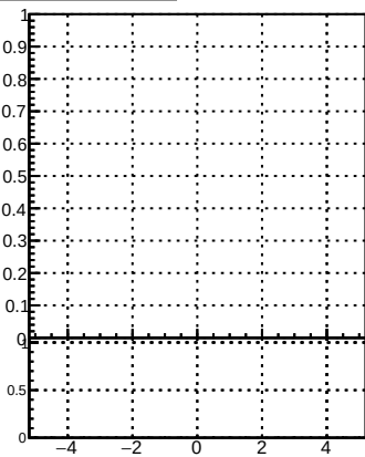
p_offset_eta_npv5_chm
