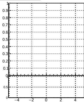
p_offset_eta_npv5_chu
