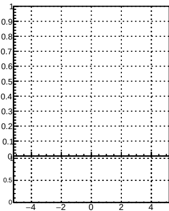
p_offset_eta_npv5_lep
