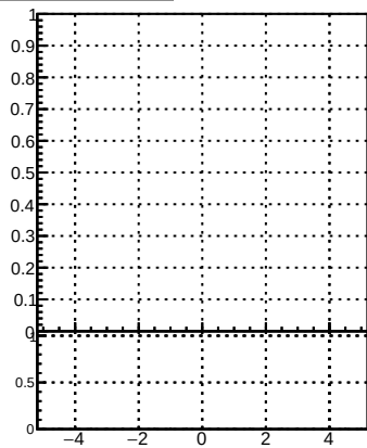
p_offset_eta_npv5_hfe
