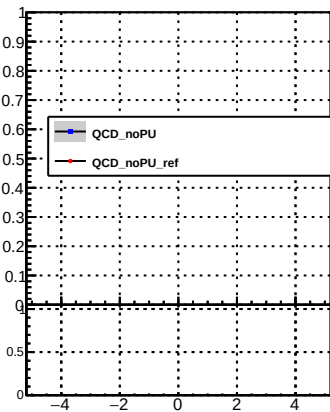
p_offset_eta_npv5_nh
