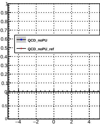
p_offset_eta_npv56_nh
