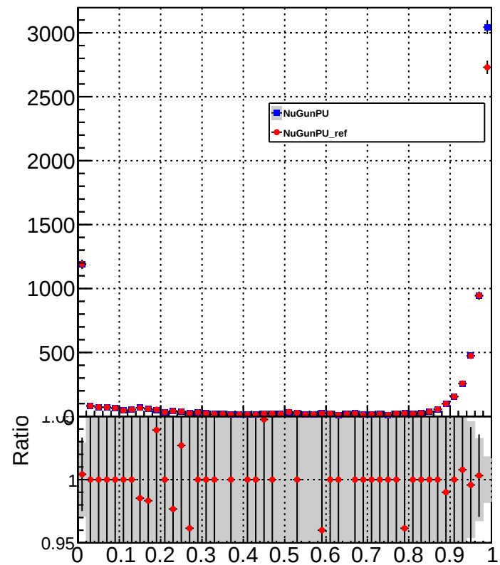
HFHadronEnergyFraction
