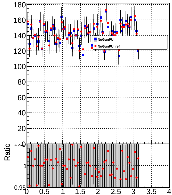
METDeltaPhi_GenMETTrue
