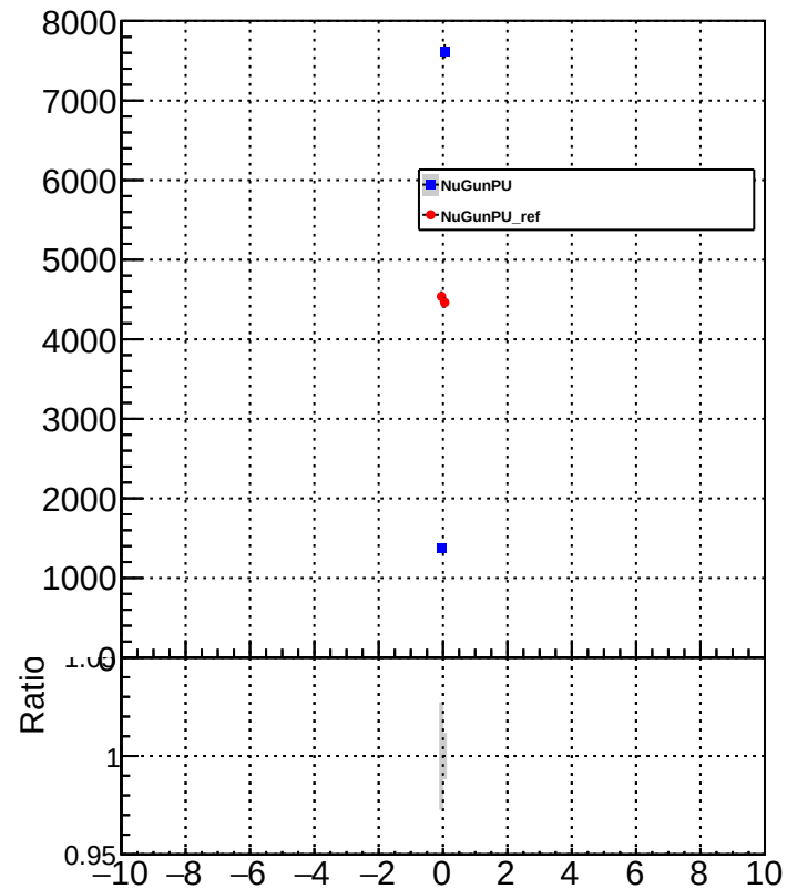
METUnc_MuonEnUp
