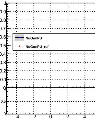
p_offset_eta_npv21_nh
