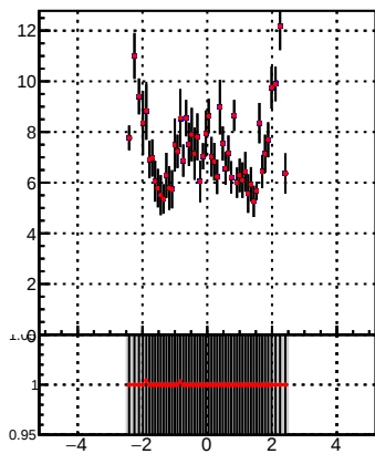
p_offset_eta_npv27_chm
