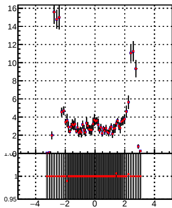
p_offset_eta_npv27_chu
