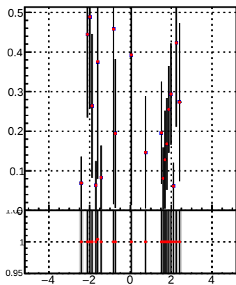
p_offset_eta_npv27_lep
