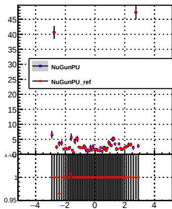
p_offset_eta_npv27_nh
