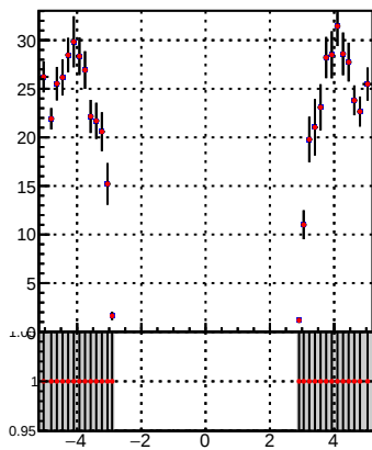
p_offset_eta_npv27_hfh
