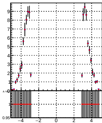
p_offset_eta_npv27_hfe
