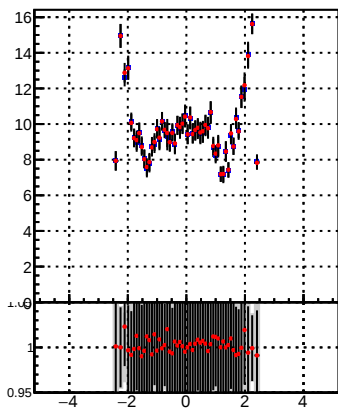
p_offset_eta_npv31_chm
