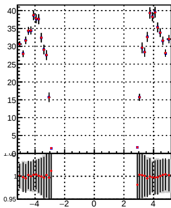
p_offset_eta_npv31_hfh
