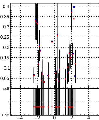
p_offset_eta_npv31_lep
