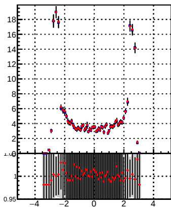
p_offset_eta_npv31_chu
