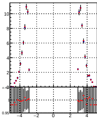
p_offset_eta_npv31_hfe
