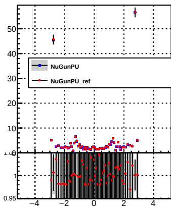
p_offset_eta_npv31_nh
