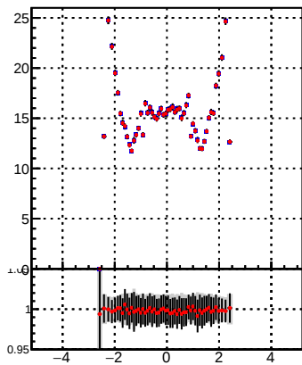
p_offset_eta_npv52_chm
