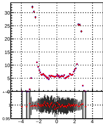
p_offset_eta_npv52_chu
