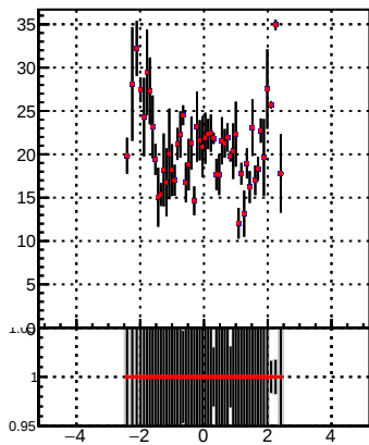
p_offset_eta_npv72_chm
