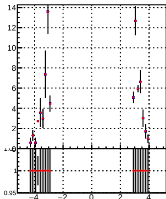
p_offset_eta_npv72_hfe
