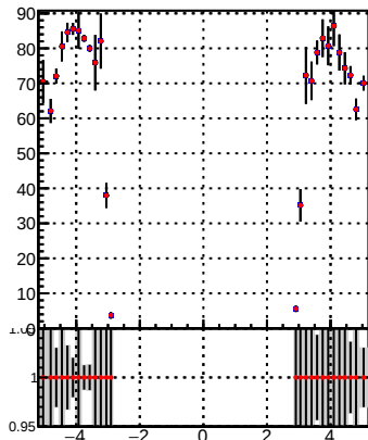
p_offset_eta_npv72_hfh
