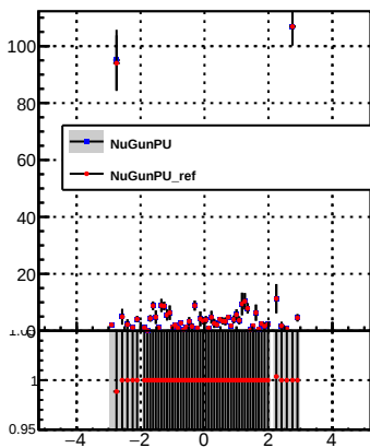
p_offset_eta_npv72_nh
