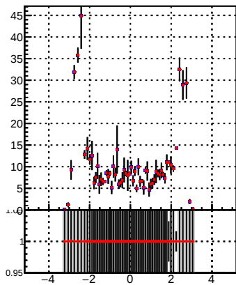
p_offset_eta_npv72_chu
