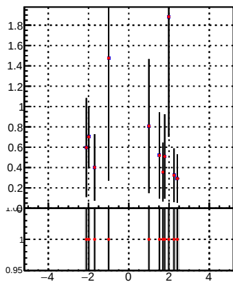
p_offset_eta_npv72_lep
