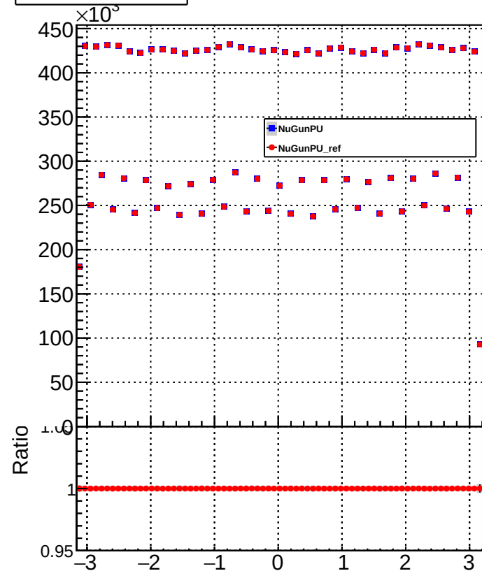
AllCandidatePhi
