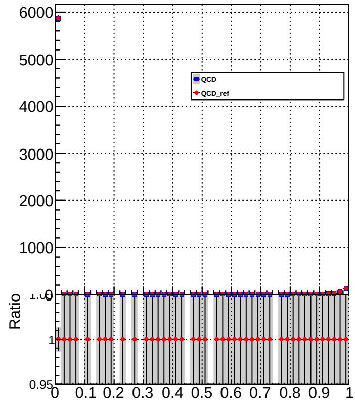
HFHadronEnergyFraction
