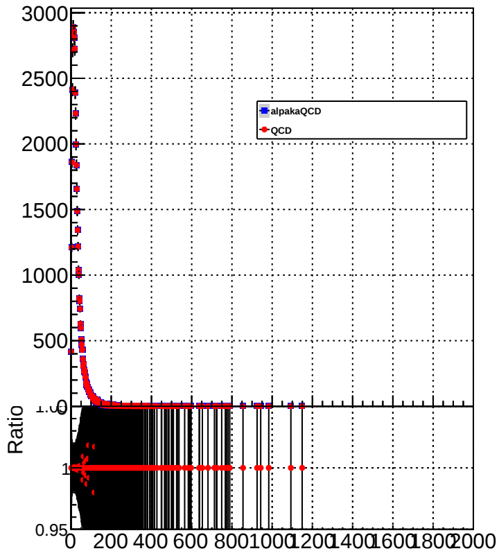
MET (2 GeV binning)
