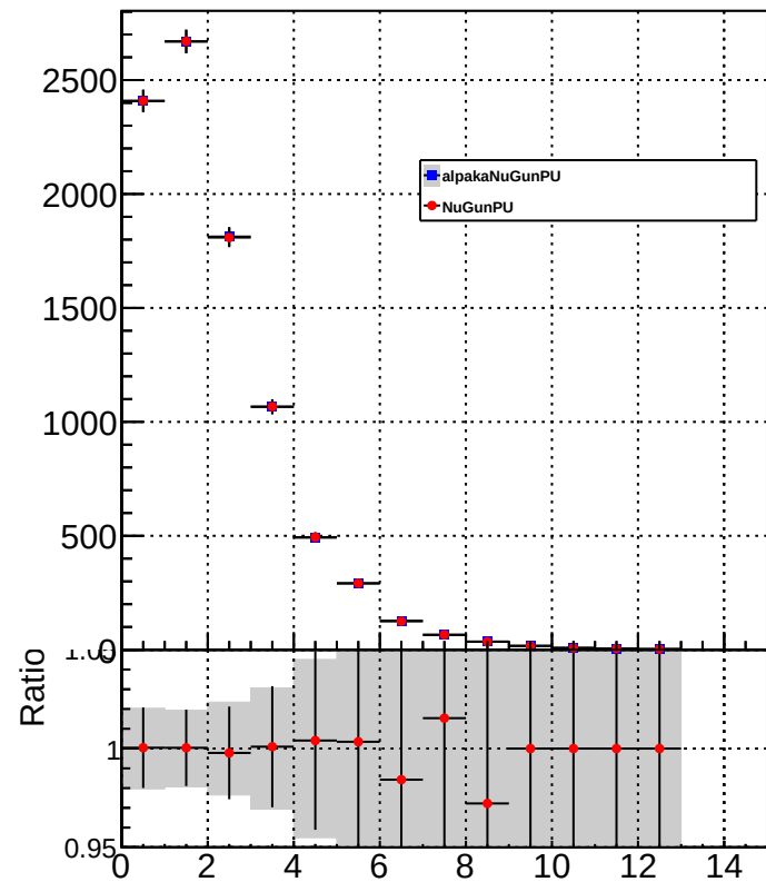
NJetsEta_B 20<Pt<40
