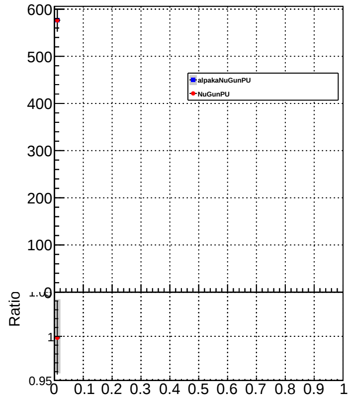
HFEMEnergyFraction
