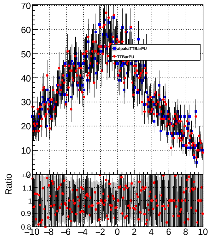
METUnc_JetResUp
