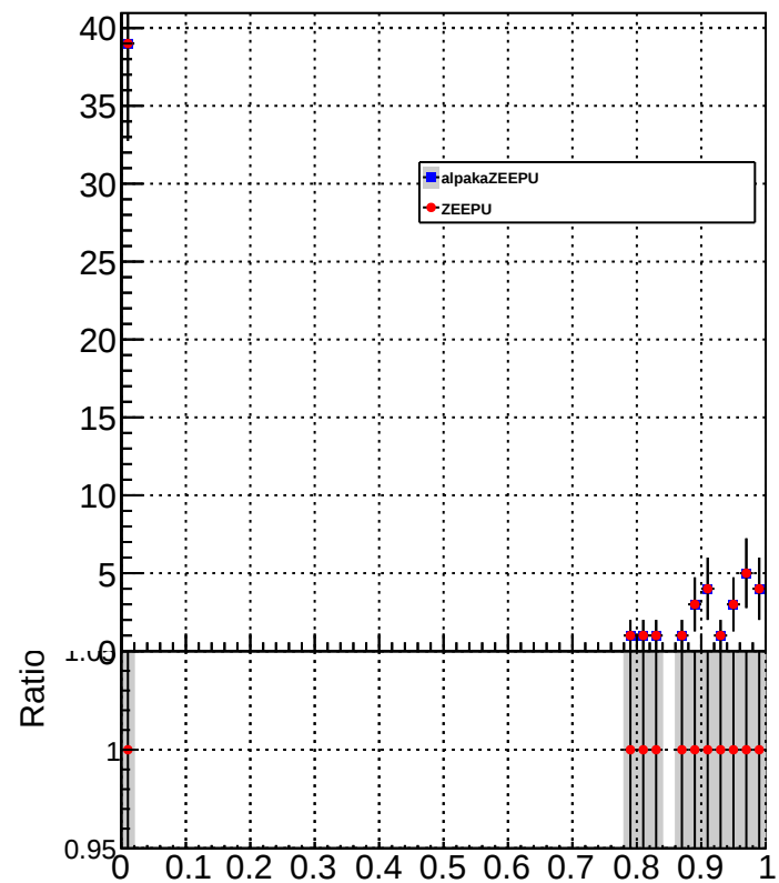
chargedEmEnergyFraction
