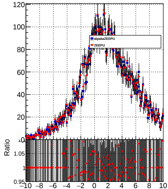
METUnc_JetEnDown
