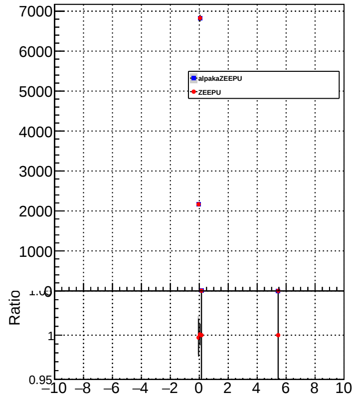
METUnc_MuonEnDown
