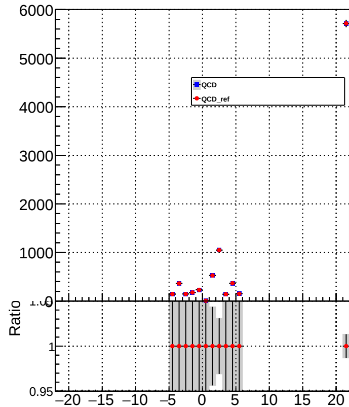
PartonFlavor
