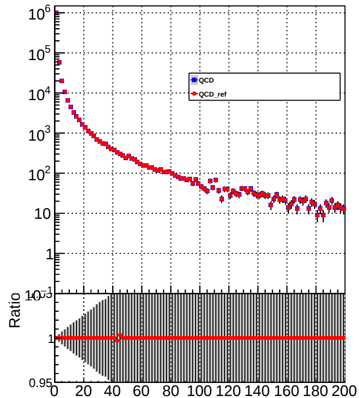
AllCandidatePtMid
