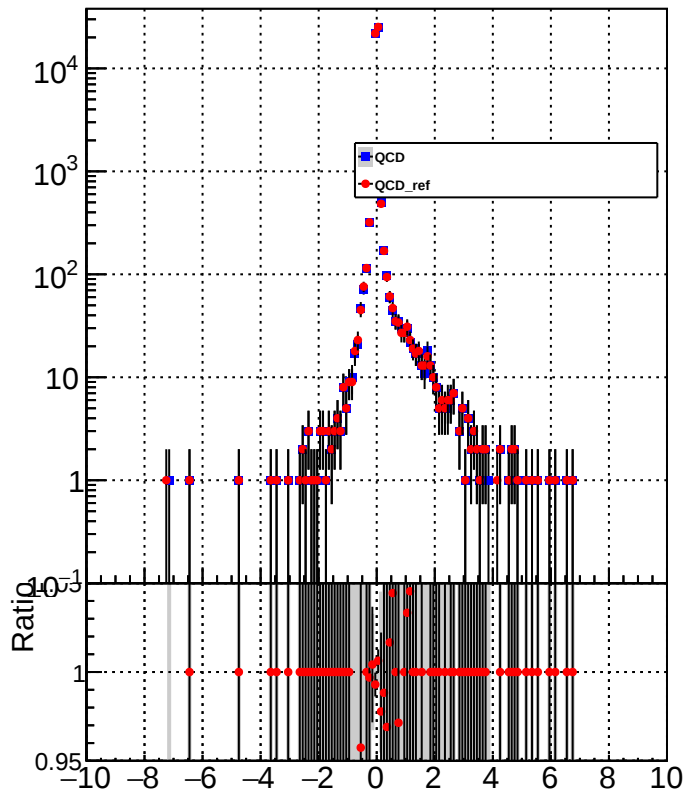
METUnc_ElectronEnDown
