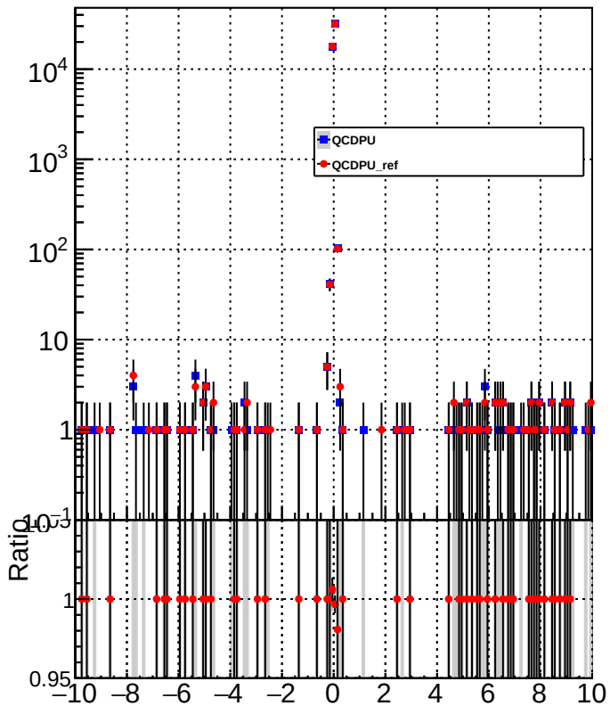
METUnc_MuonEnUp
