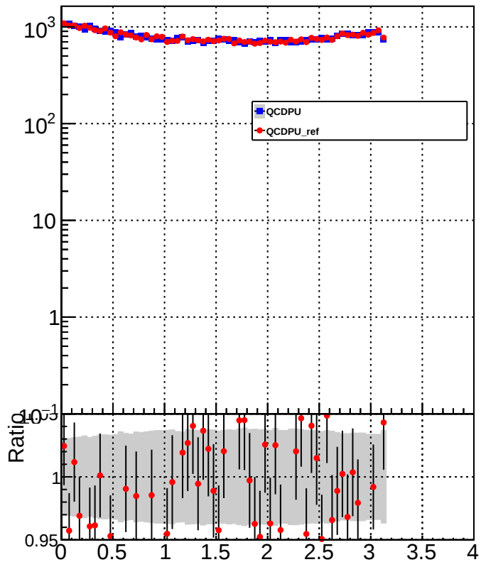
METDeltaPhi_GenMETTrue
